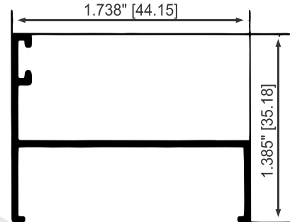
BATIENTE LATERAL ECONÓMICA 5056
