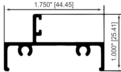
BATIENTE SUPERIOR PARA PUERTA DE 1" 5041
